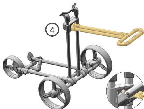
Handle in Position bringen und ggf. einstellen. Niedrigeres Handel: Haken gegen Uhrzeigersinn drehen. Höheres Handel: Haken im Uhrzeigersinn drehen.
